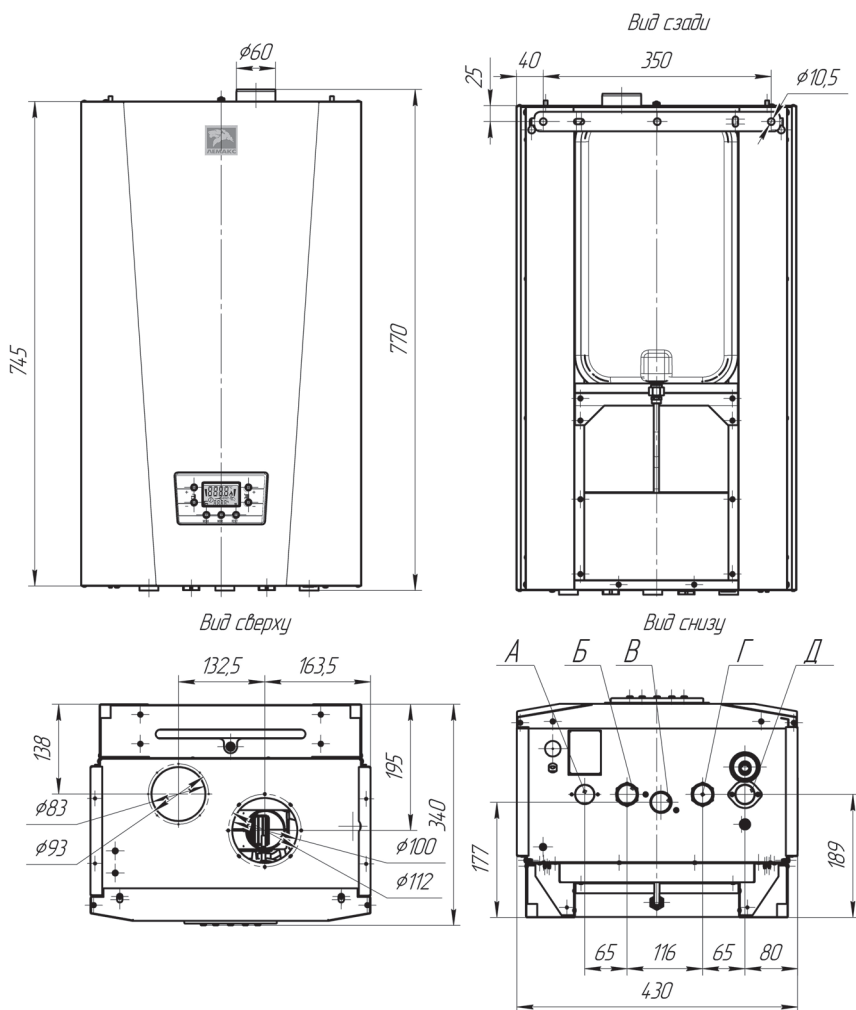
Рис 2.2. Габаритные и присоединительные размеры котлов PRIME-V26,28,32 NO
