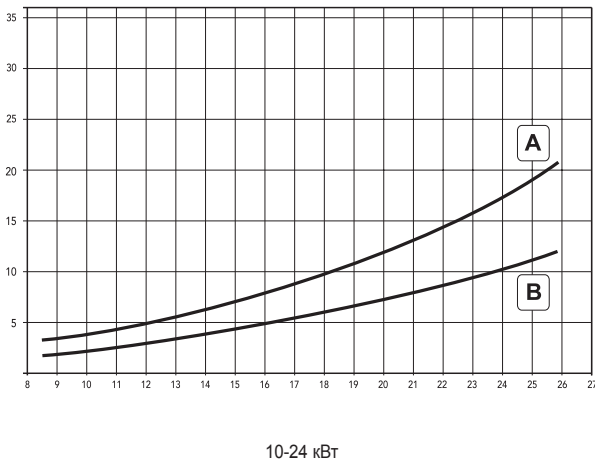
Рис. 16. Кривая давление газа/мощность: А – сжиженный газ; В – метан
