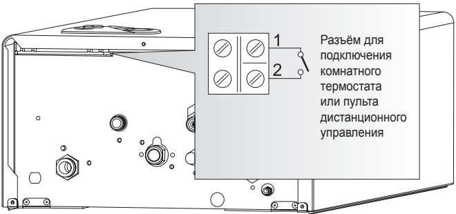
Рис. 5. Доступ к клеммной колодке
