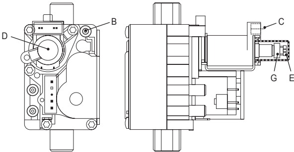
Рис. 12. Газовый клапан
